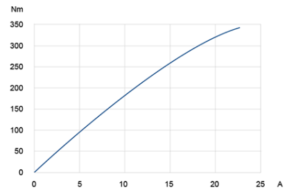
Grafico assorbimento/coppia
