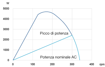
Grafico velocità/potenza
