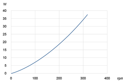
Perdite rotore
