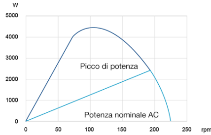
Grafico velocità/potenza
